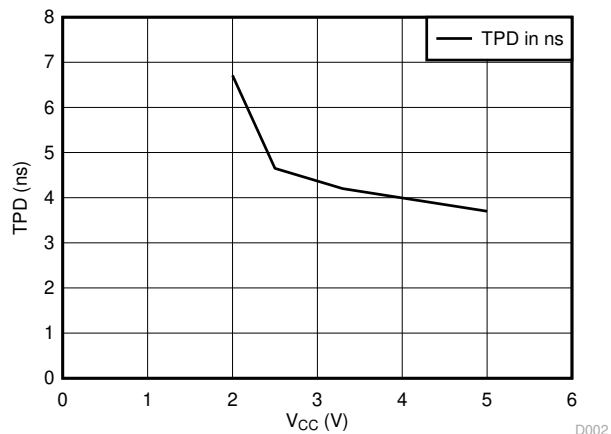
图 5-3. TPD vs VCC
