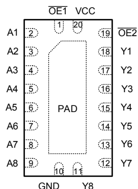
图 4-1. SN74AHC540-Q1 RKS 封装 (顶视图)
