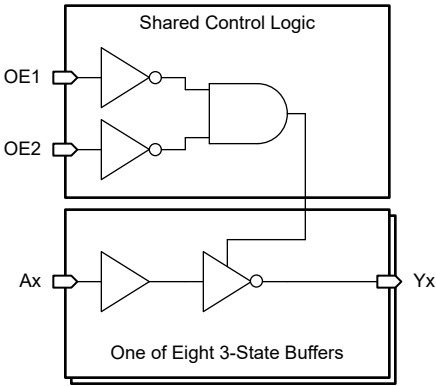
功能方框图
