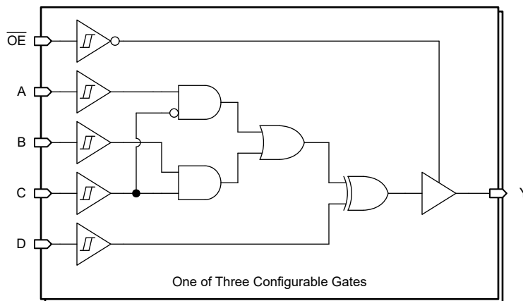
功能方框图
