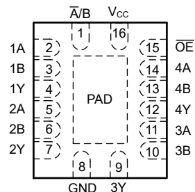
图 5-2. WBQB 封装，16 引脚 WQFN（透明顶视图）
