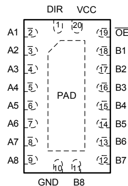
图 4-2. SN74AHC245-Q1 WRKS 封装，20 引脚 WQFN（顶视图）
