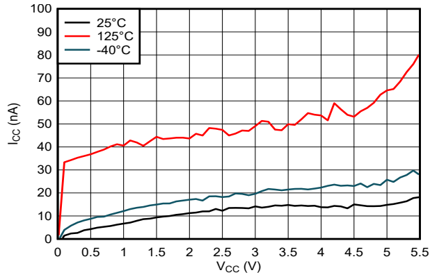
图 5-1. 电源电流与电源电压之间的关系
