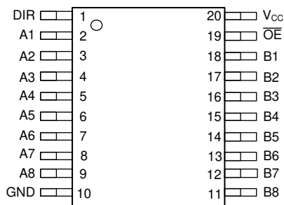
图 4-1. SN74AHC245-Q1 PW 或 DGS 封装，20 引脚 TSSOP 或 VSSOP（顶视图）
