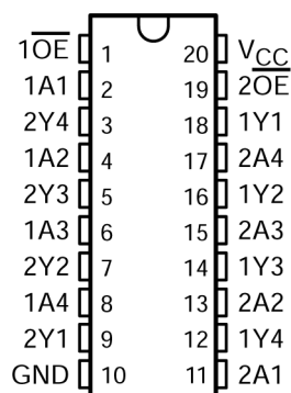
图 5-1. DW or PW Package (Top View)
