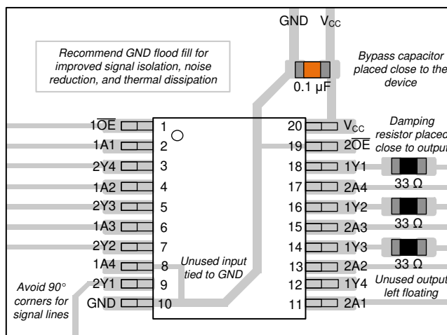
图 7-1. Layout Diagram
