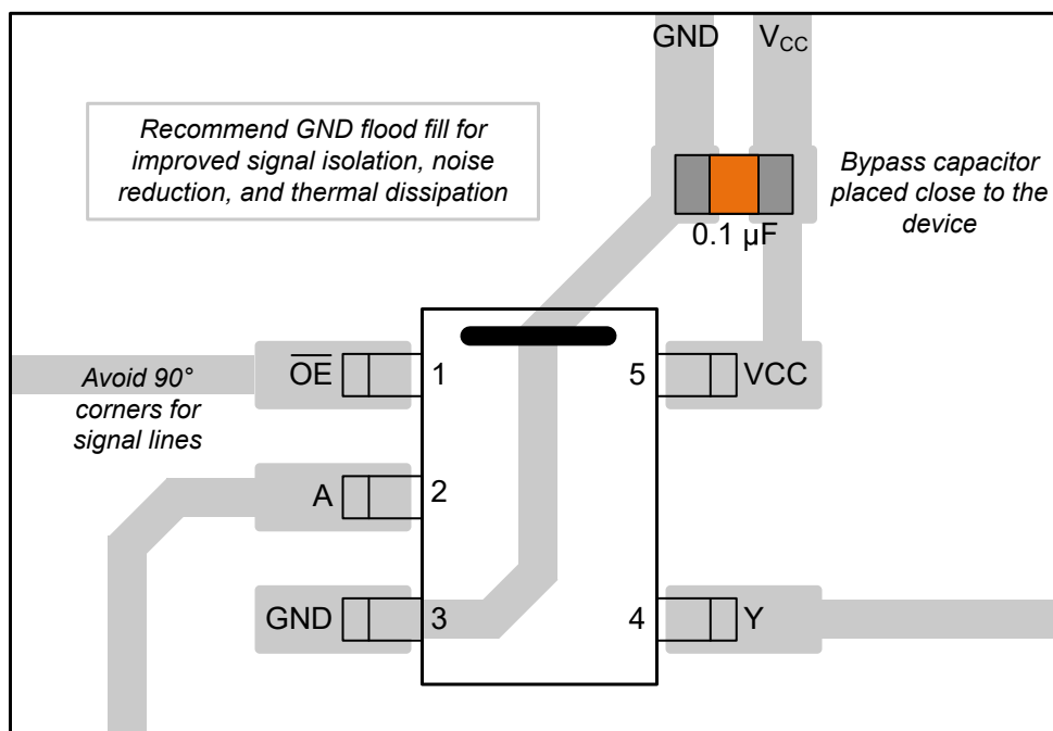
图 11-1. SN74AHC1G125-Q1 的示例布局
