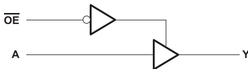
简化逻辑图 (正逻辑)
