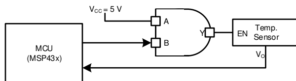
图 9-1. 典型应用图
