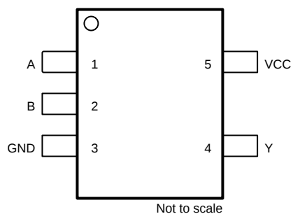
图 5-1. DBV 或 DCK 封装，5 引脚 SOT-23 或 SC70 (顶视图)
