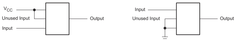
图 9-3. 布局图
