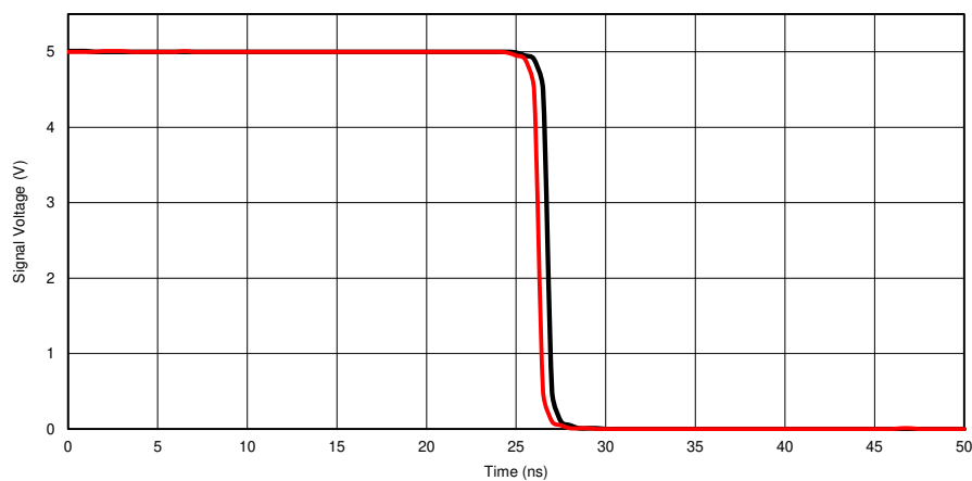
图 6-1. 25°C 时 TPD 与 V_{CC} 间的关系
