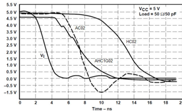
图 9-2. 应用曲线
