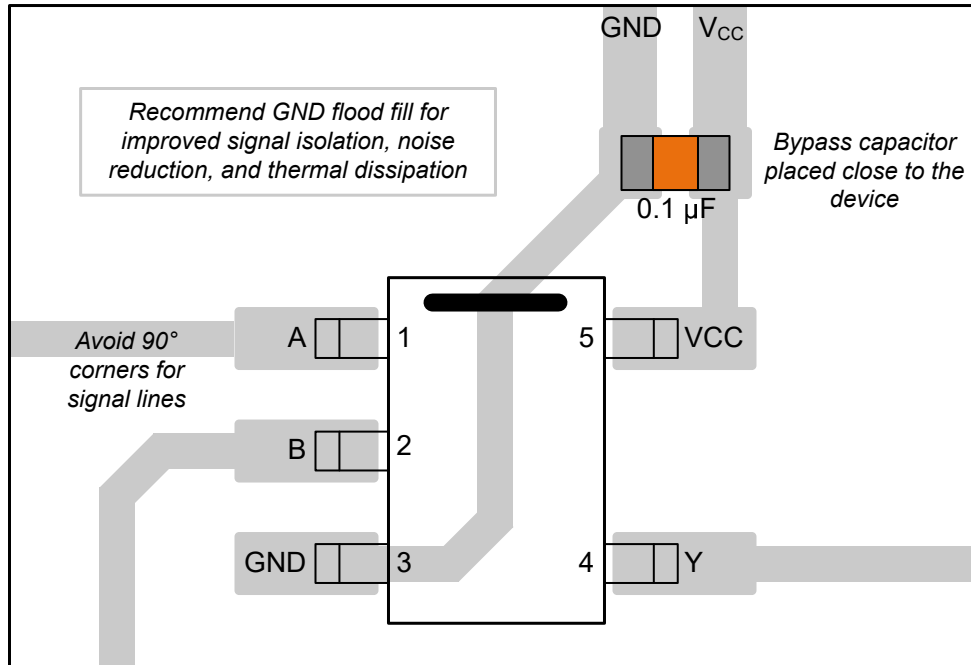
图 9-3. SN74AHC1G02-Q1 的示例布局
