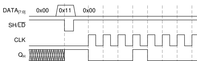
图 8-2. 应用时序图
