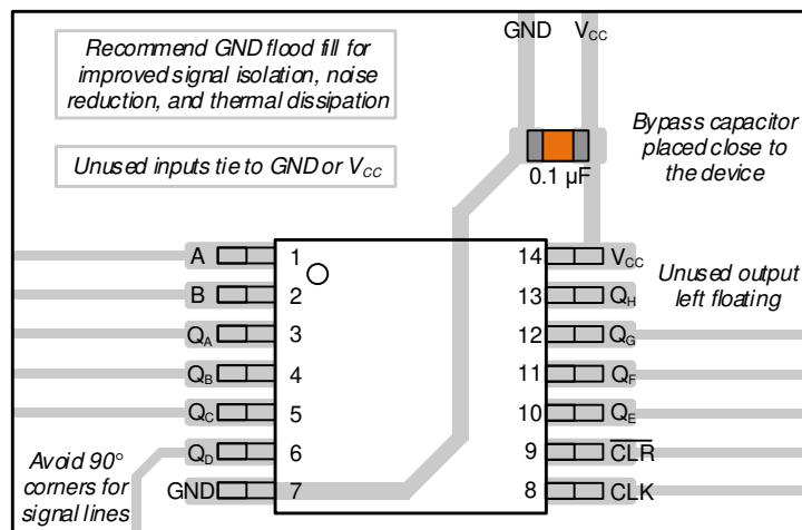
图 8-3. SN74AHC164 的示例布局
