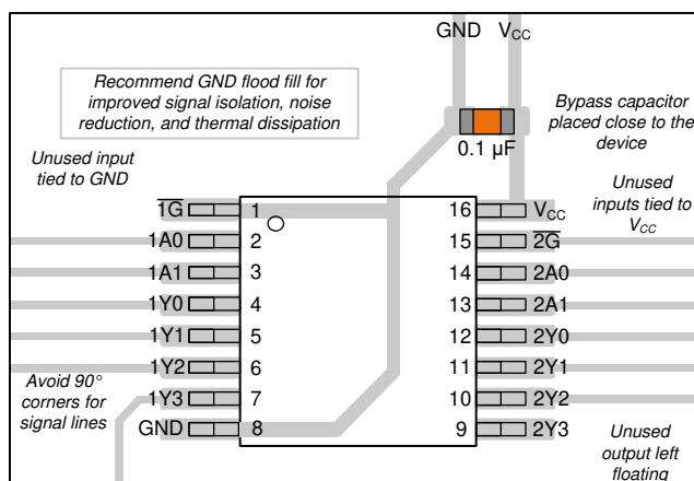
图 8-3. SN74AHC139-Q1 的示例布局
