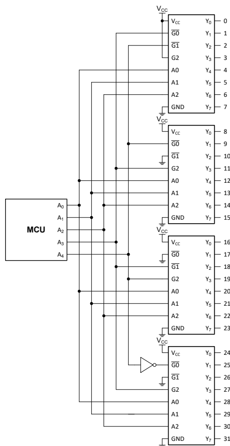
图 8-1. 典型应用框图
