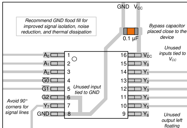
图 8-3. SN74AHC138-Q1 的示例布局
