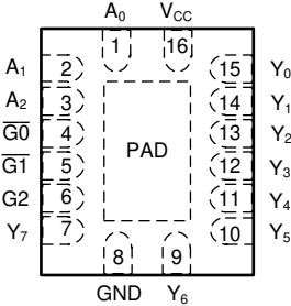
图 4-2. WBQB 封装， 16 引脚 WQFN (顶视图)
