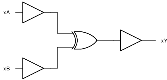
逻辑图
