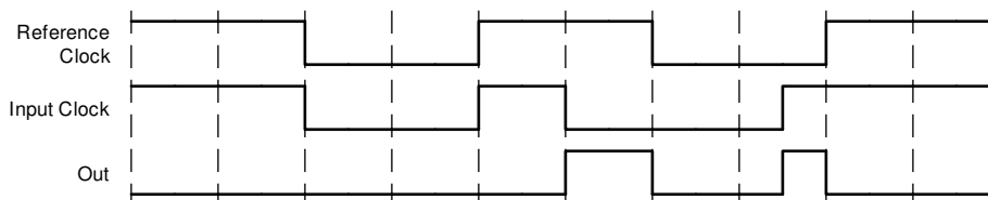
图 8-2. 应用时序图
