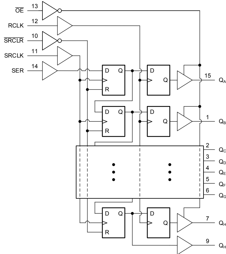
功能图
