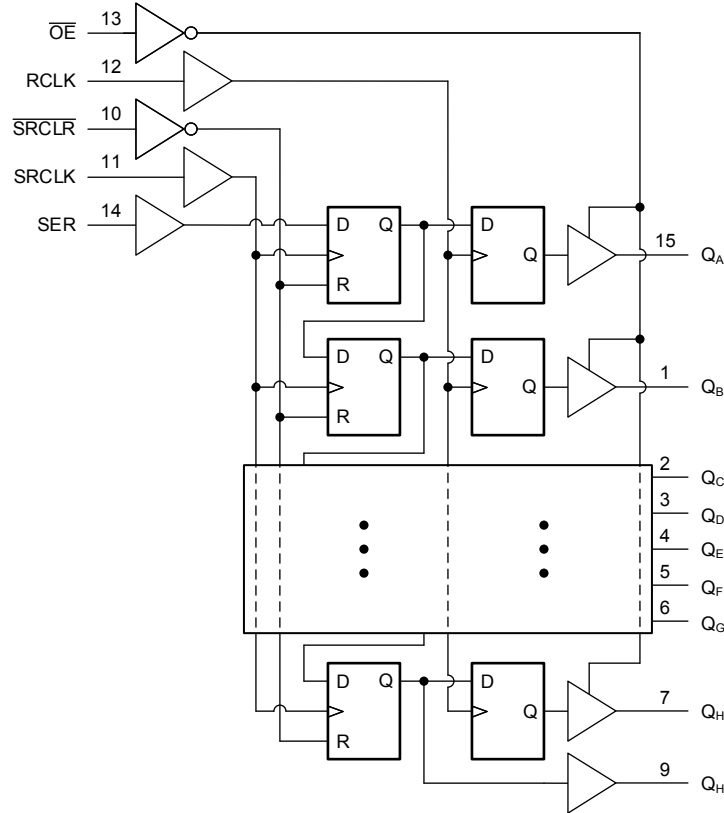
图 7-1. SN74ACT595 的逻辑图 (正逻辑)
