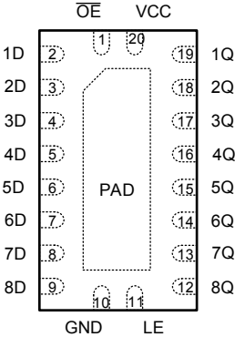
图 4-2. SN74ACT573-Q1 RKS 封装，20 引脚 VQFN (顶视图)
