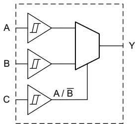
2 线至 1 线数据选择器
