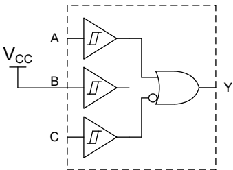
具有 1 个反相输入的双输入或门
