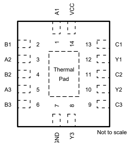
图 4-2. SN74ACT3G97-Q1 BQA 封装，14 引脚 WQFN (顶视图)
