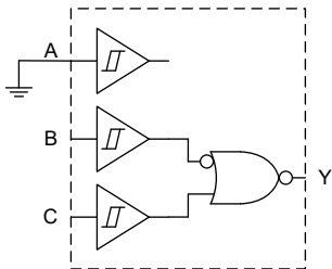
具有 1 个反相输入的双输入或非门
