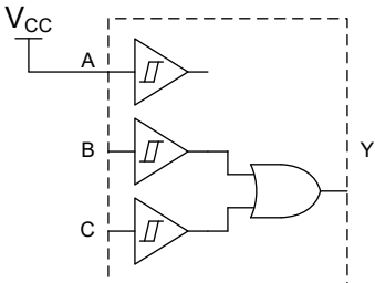
双输入或门
