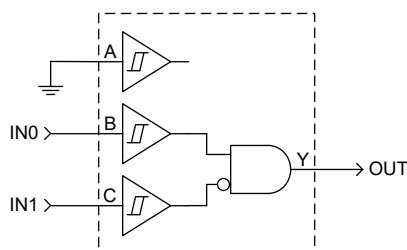
图 8-1. 典型应用原理图
