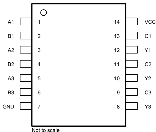
图 4-1. SN74ACT3G97-Q1 PW 封装，14 引脚 TSSOP (顶视图)
