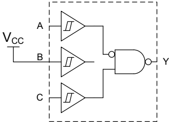
具有 1 个反相输入的双输入与非门
