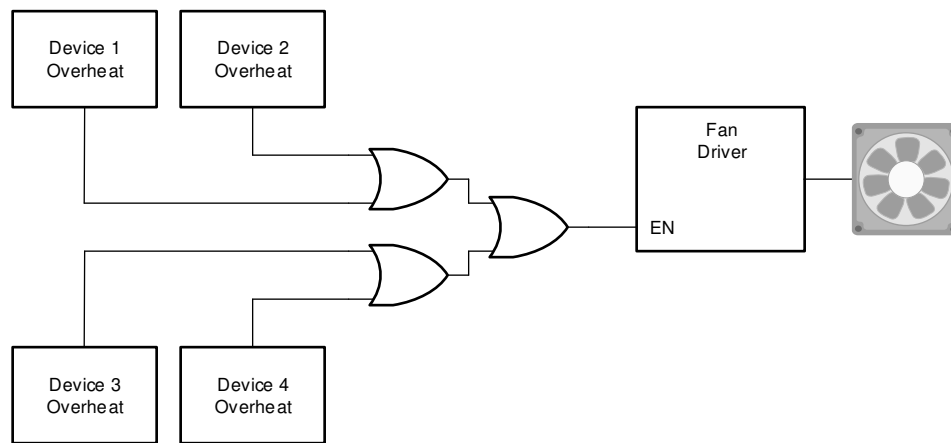
图 8-1. 典型应用原理图
