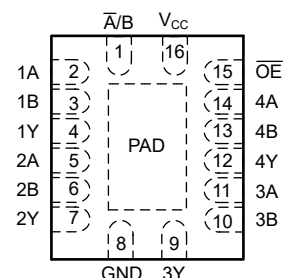
图 4-2. BQB 封装，16 引脚 WQFN（透明顶视图）
