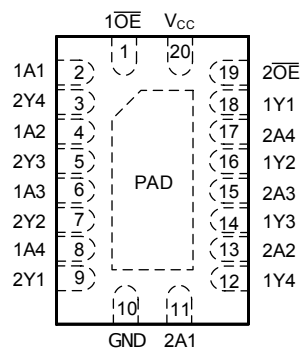
图 4-2. SN74ACT240-Q1 VQFN 封装 (顶视图)
