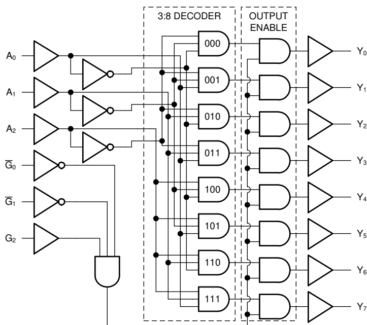
图 7-1. SN74ACT238-Q1 的逻辑图 (正逻辑)
