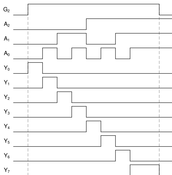
图 8-2. 应用时序图
