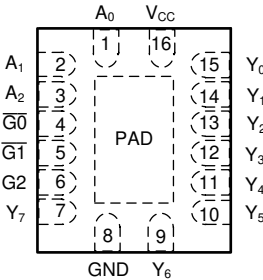
BQB 封装，16 引脚 WQFN（透明顶视图）
