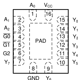
BQB 封装，16 引脚 WQFN (透明顶视图)
