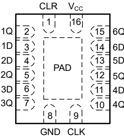
BQB 封装，16 引脚 TSSOP（透明顶视图）
