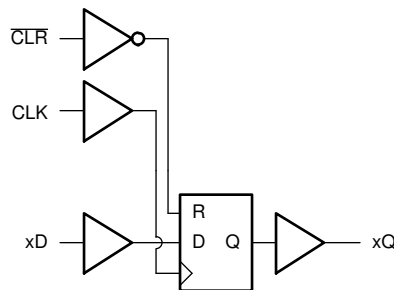
功能图
