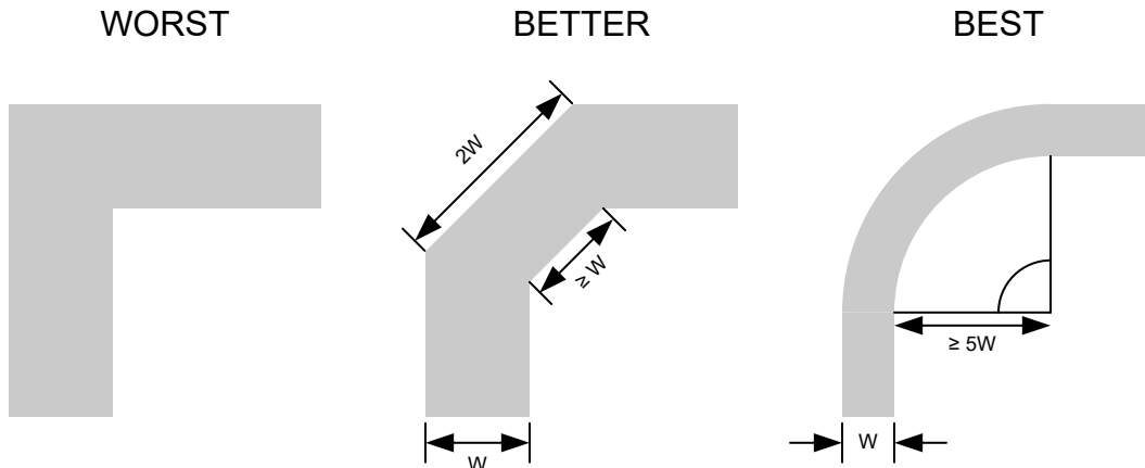
图 8-1. 可改善信号完整性的布线转角示例
