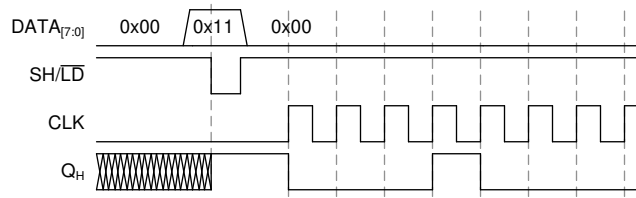
图 8-2. 应用时序图
