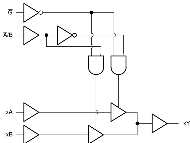
图 7-1. SN74ACT157-Q1 的逻辑图 (正逻辑)
