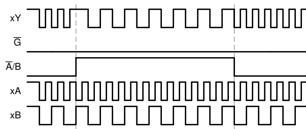
图 8-2. 应用时序图
