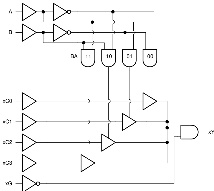
图 7-1. SN74ACT153-Q1 的逻辑图 (正逻辑)
