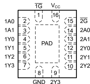
BQB 封装，16 引脚 WQFN（透明顶视图）
