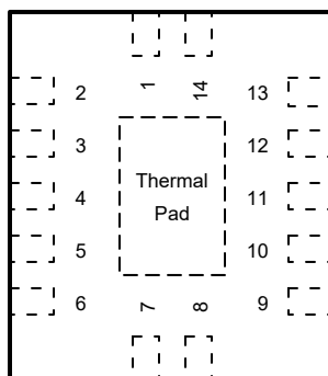
图 4-1. SN74ACT11-Q1 BQB 封装 (透明顶视图)
