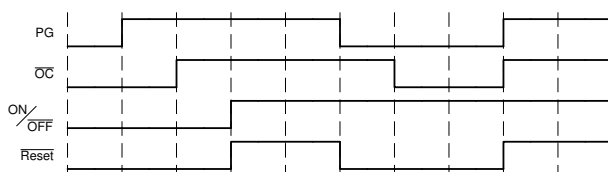
图 8-2. 典型应用时序图
