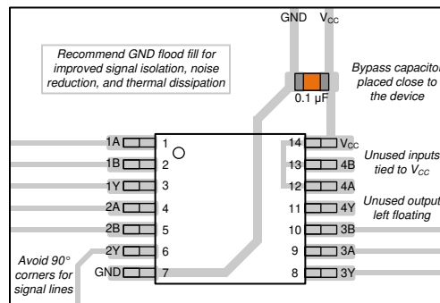
图 8-3. SN74ACT08-Q1 的示例布局
