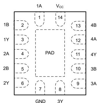
BQA 封装 14 引脚 WQFN 俯视图
