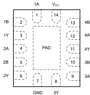
图 3-3. BQA 封装（顶视图）
