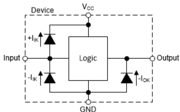
图 7-3. 每个输入和开漏输出的钳位二极管的电气布置
