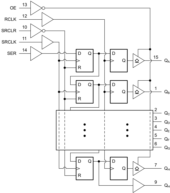
功能图
