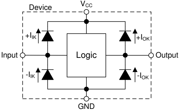
图 7-3. 每个输入和推挽输出的钳位二极管的电气布置
