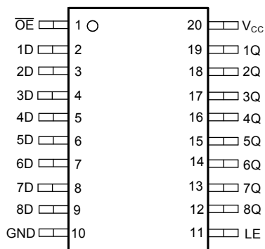
图 4-1. SN74AC573-Q1 DGS 或 PW 封装，20 引脚 VSSOP 或 TSSOP (顶视图)
