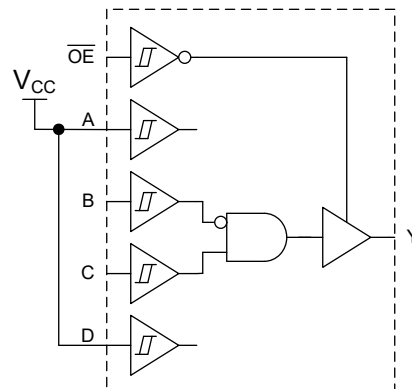
具有 1 个反相输入的双输入与门
