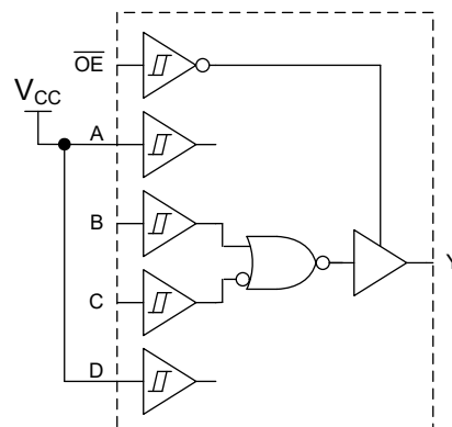
具有 1 个反相输入的双输入或非门
