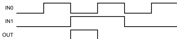
图 8-2. 典型应用时序图
