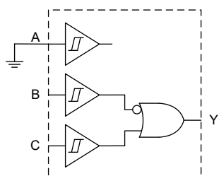
具有 1 个反相输入的双输入或门
