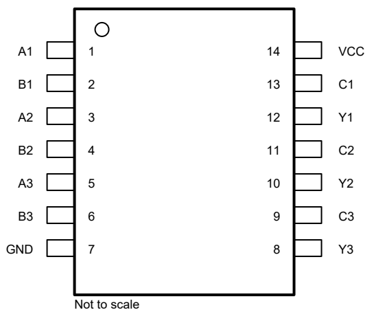
图 4-1. SN74AC3G97-Q1 PW 封装 ( 预发布 ) , 14 引脚 TSSOP ( 顶视图 )
