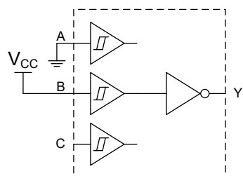
施密特触发反相器
