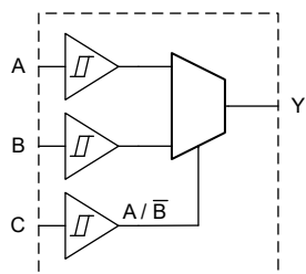
2 线至 1 线数据选择器
