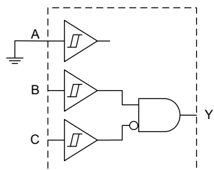
具有 1 个反相输入的双输入与门
