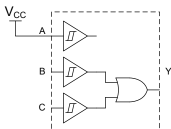
双输入或门
