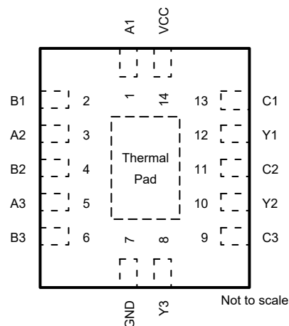
图 4-2. SN74AC3G97-Q1 BQA 封装 , 14 引脚 WQFN ( 顶视图 )
