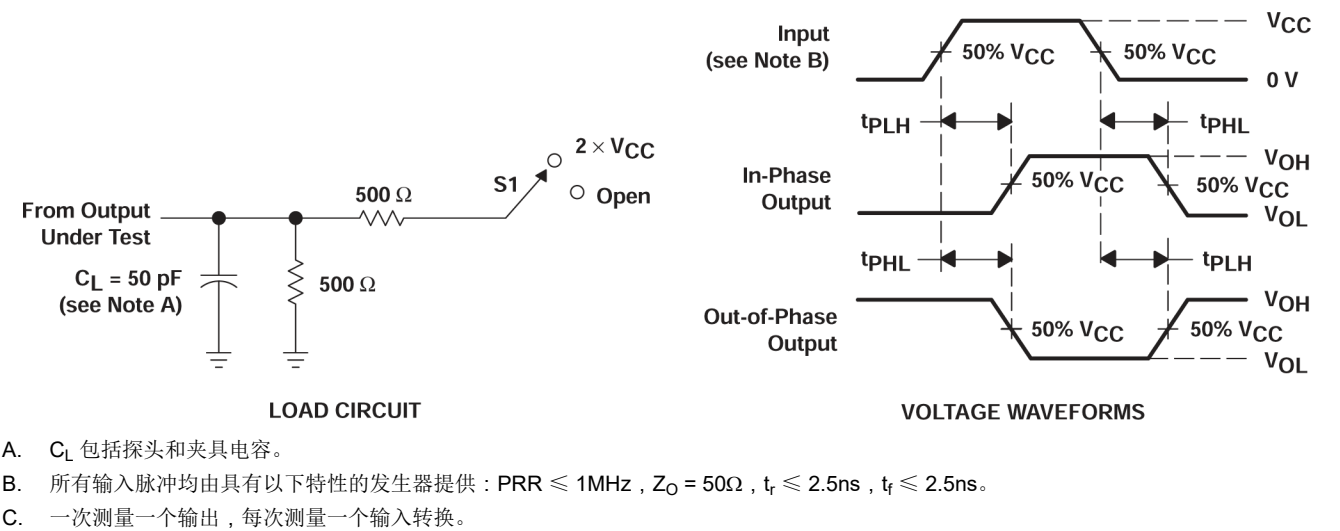
图 5-1. 负载电路和电压波形
