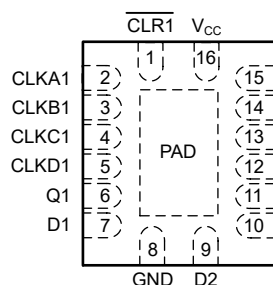
图 4-1. BQB 封装，16 引脚 WQFN（顶视图）
