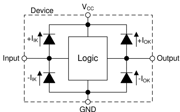
图 7-10. 每个输入和输出的钳位二极管的电气布置
