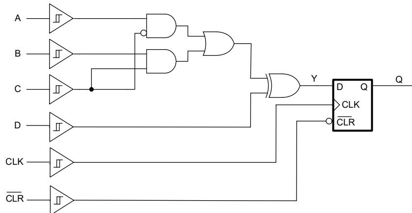
逻辑图（正逻辑）
