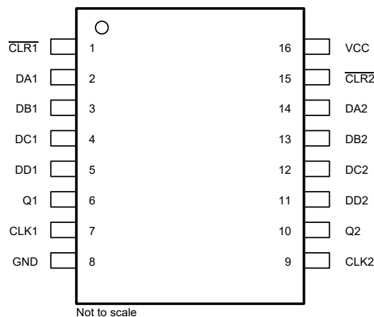
图 4-2. PW 封装，16 引脚 TSSOP（预发布）（顶视图）
