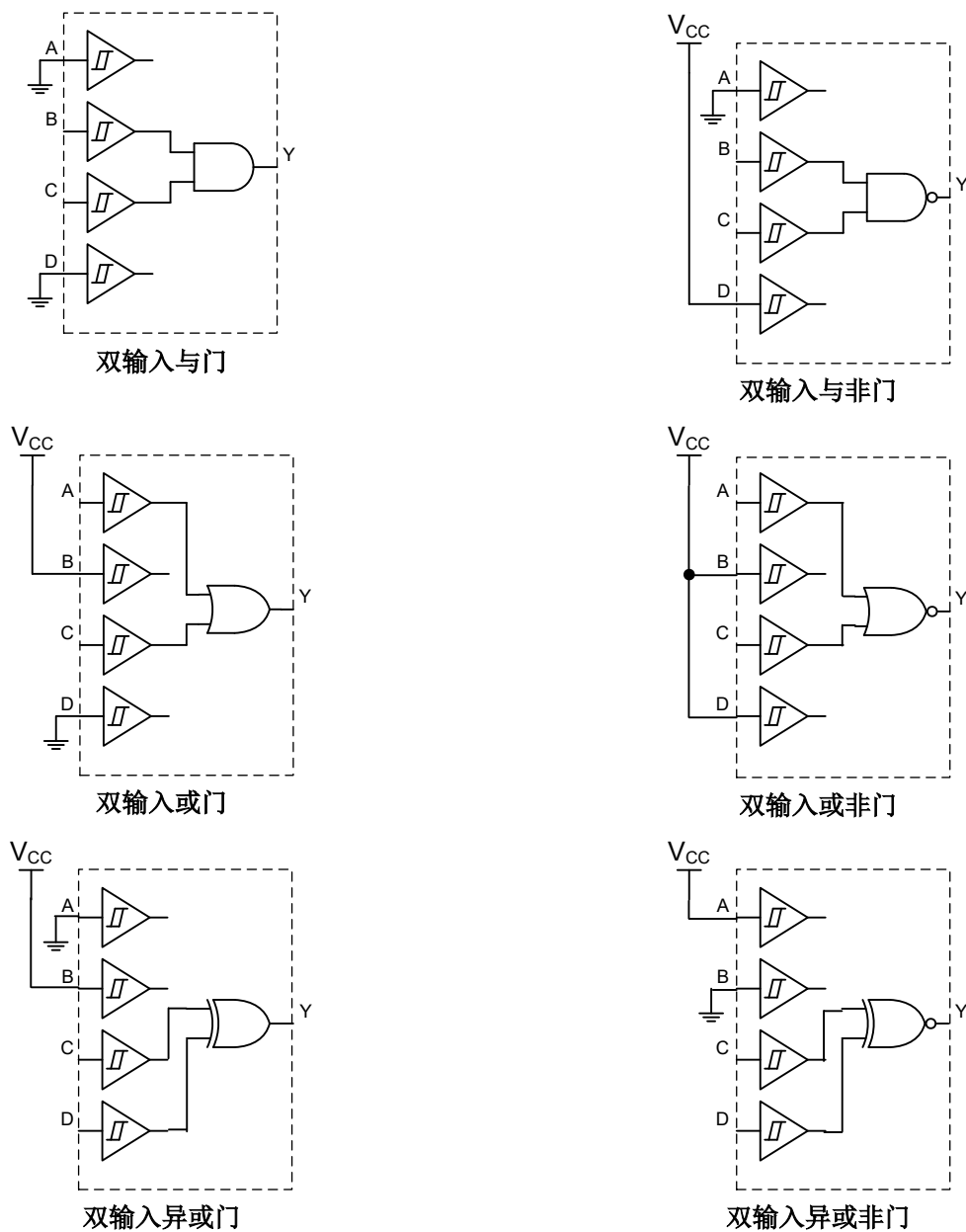
图 7-3. 逻辑配置
