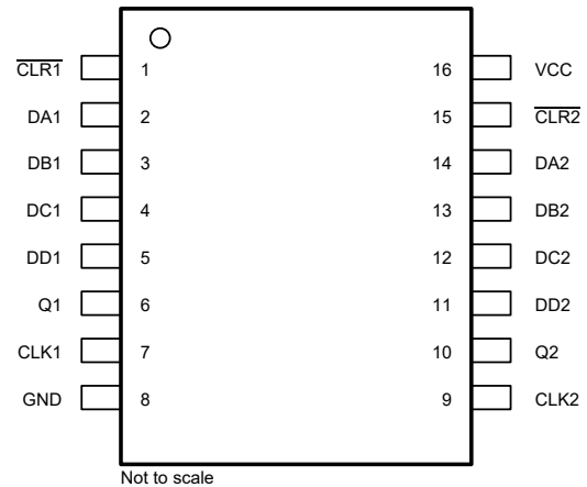
图 4-2. PW 封装，16 引脚 TSSOP（顶视图）
