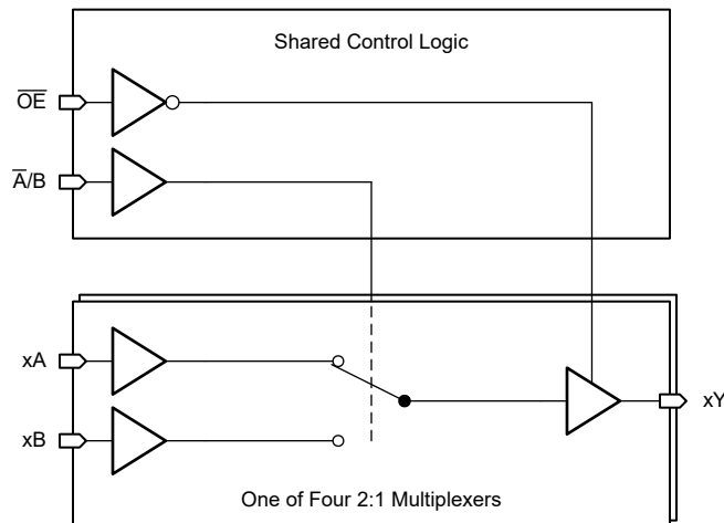
逻辑图
