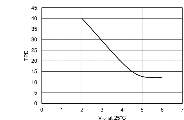
图 5-1. TPD vs V_{CC} at 25^\circ\text{C}
