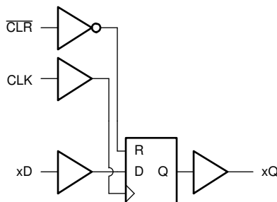
图 7-1. SN74ACT164-Q1 的逻辑图 (正逻辑)
