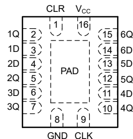
BQB 封装，16 引脚 TSSOP (透明顶视图)
