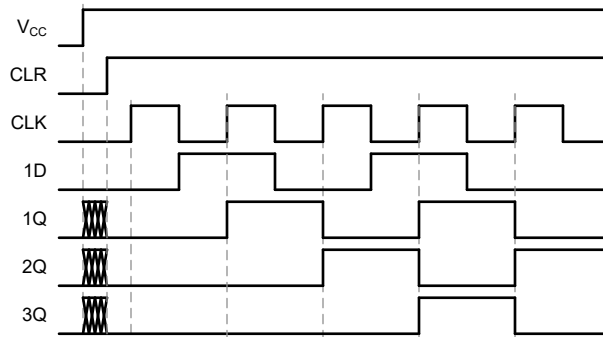
图 8-2. 应用时序图
