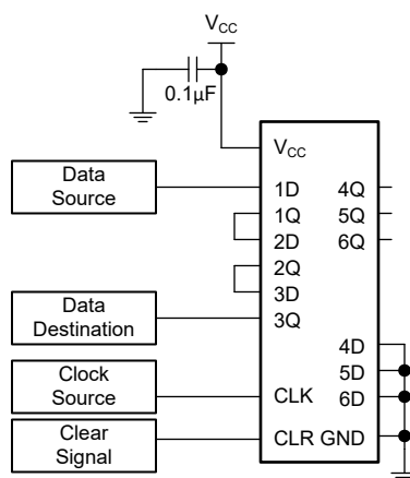
图 8-1. 典型应用框图
