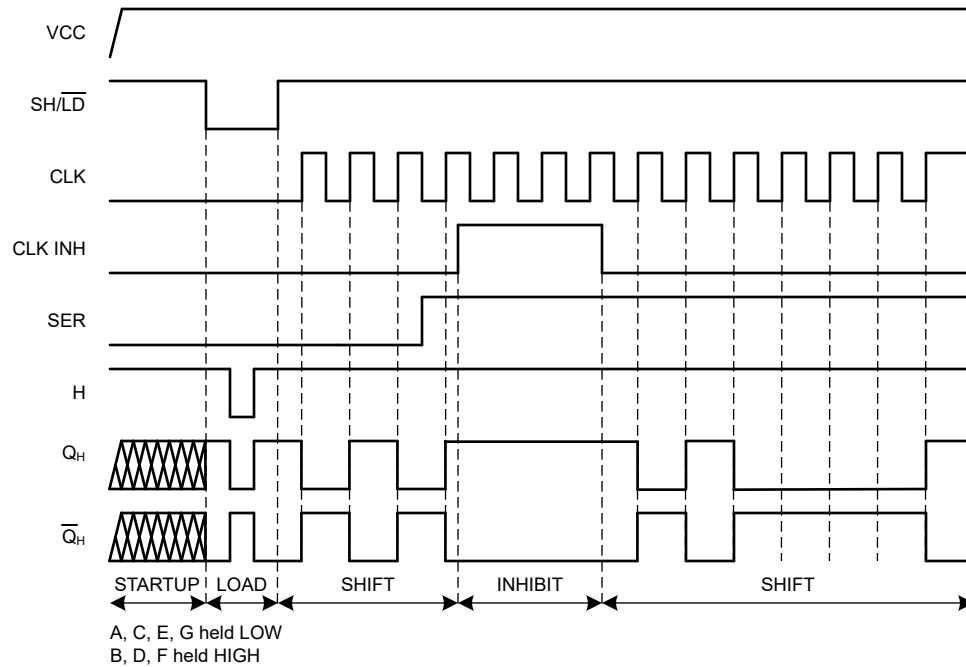
图 5-1. 时序图
