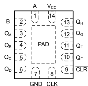
图 4-2. WBQA 封装 14 引脚 WQFN (顶视图)
