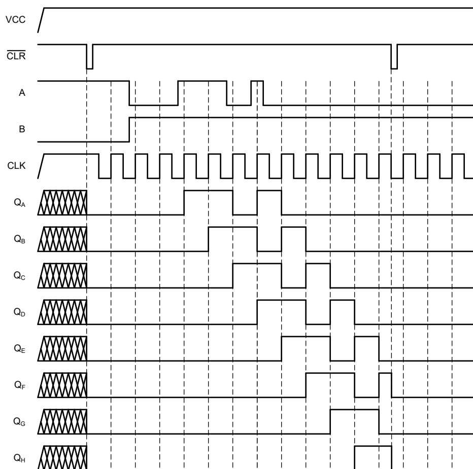
图 5-1. 时序图
