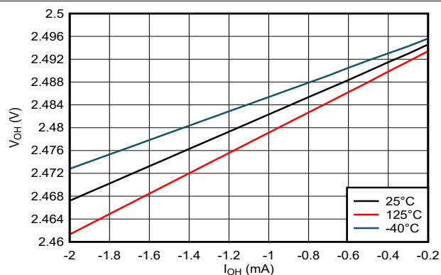
图 5-11. 高电平状态下输出电压与电流间的关系 (2.5V 电源)
