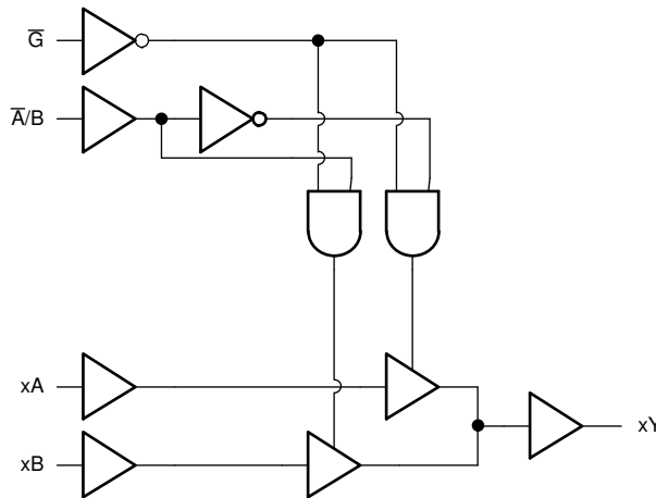
图 7-1. SN74AC157-Q1 的逻辑图 (正逻辑)
