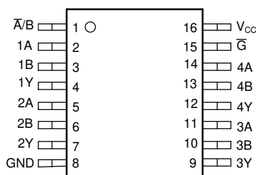
图 4-1. PW 封装，16 引脚 TSSOP (俯视图)
