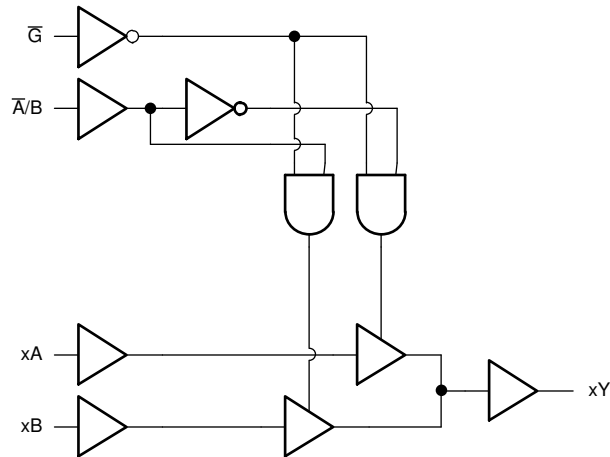
逻辑图
