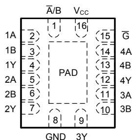
图 4-2. BQB 封装，16 引脚 WQFN (俯视图)
