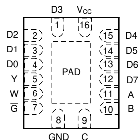
BQB 封装， 16 引脚 WQFN (透明顶视图)
