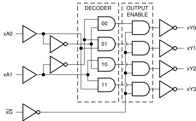
图 7-1. SN74AC139-Q1 -Q1 的逻辑图 (正逻辑)
