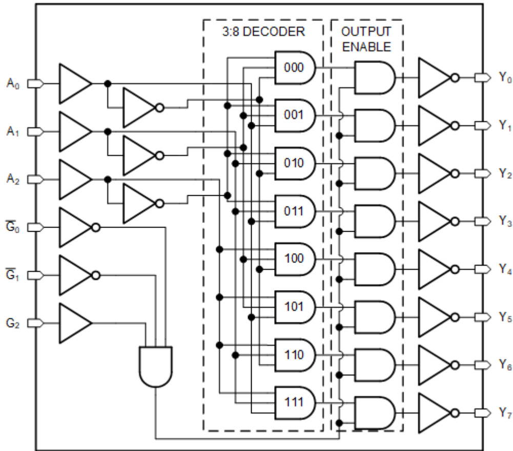
图 7-1. SN74AC138-Q1 的逻辑图 (正逻辑)
